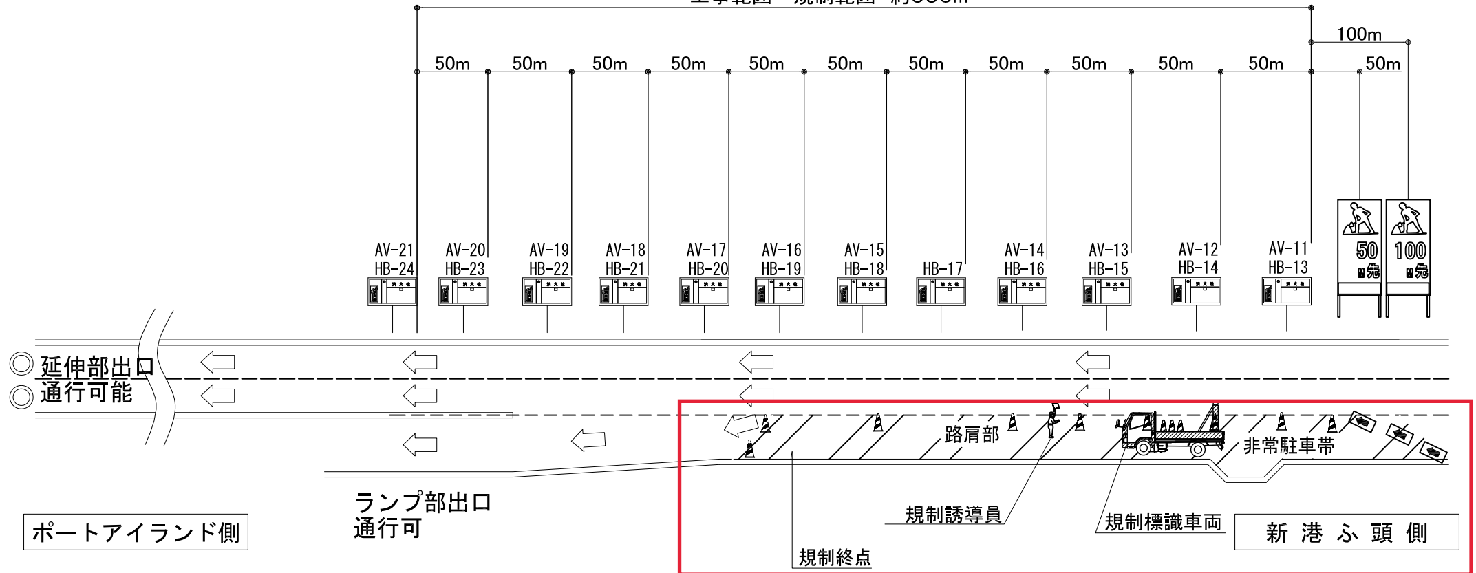
工事範囲【トンネル全体図】
